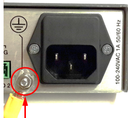
Earth stud
